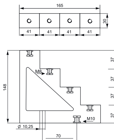
Изолятор SM "Лесенка" 600A 12кВ 4x40мм TDM
