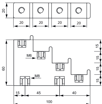
Изолятор SM "Лесенка" 300A 6кВ 4x20мм TDM
