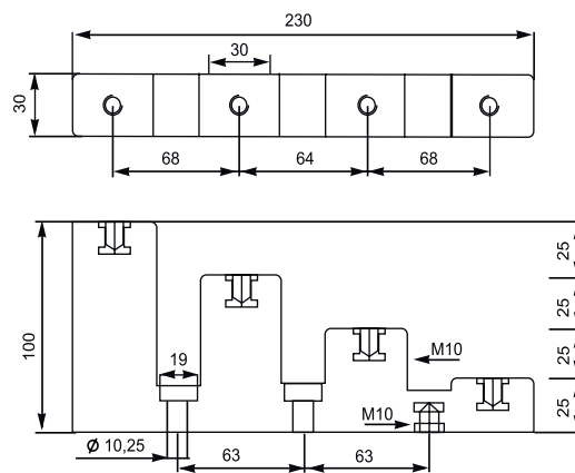
Изолятор SM "Лесенка" 900A 18кВ 4x40мм TDM
