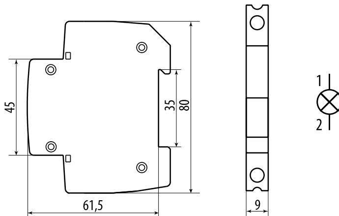
Рисунок 1. Габаритные размеры
