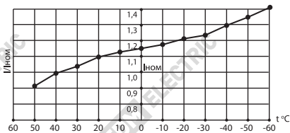
Рисунок 5. Изменение коэффициента нагрузки выключателей серии BA87 в зависимости от температуры окружающей среды. Начальная точка отсчета при I_{ном} и температуре окружающей среды +40^{\circ}\text{C} .
