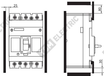
Рисунок 7. Минимальные расстояния (мм) от выключателей до металлоконструкций распределительного устройства для предотвращения перекрытия электрической дугой в процессе коммутации нагрузки.
